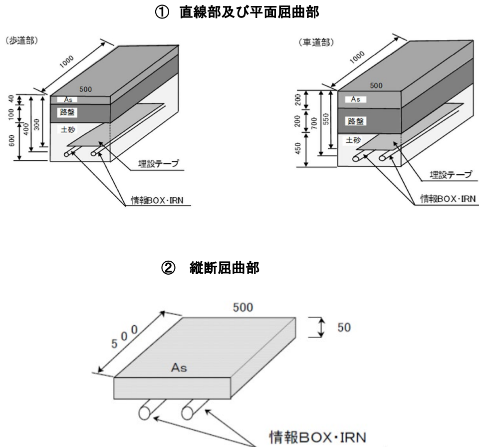
図1-1 試掘標準図
