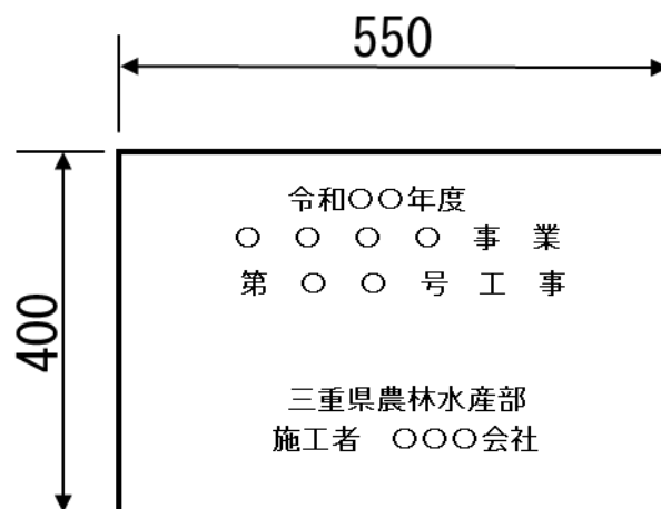
図3 施工銘板
