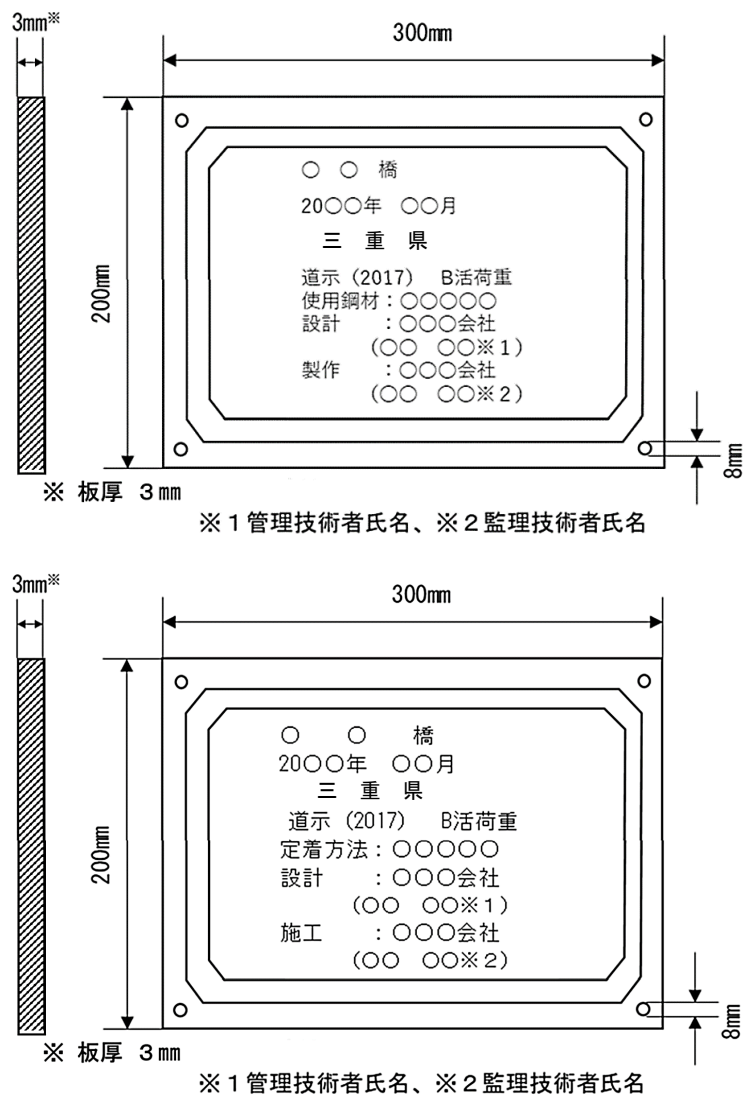
図 3-2-2 銘板の寸法及び記載事項
