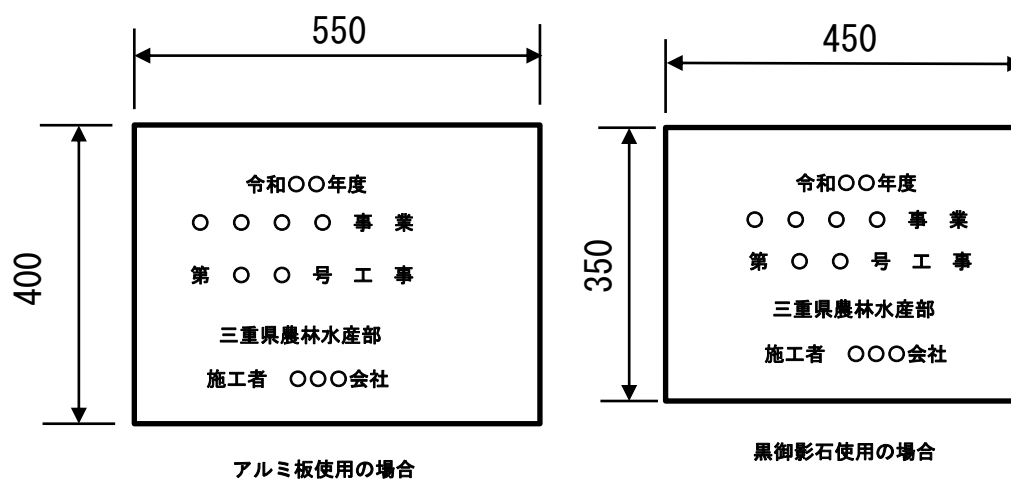
図4 施工銘板
