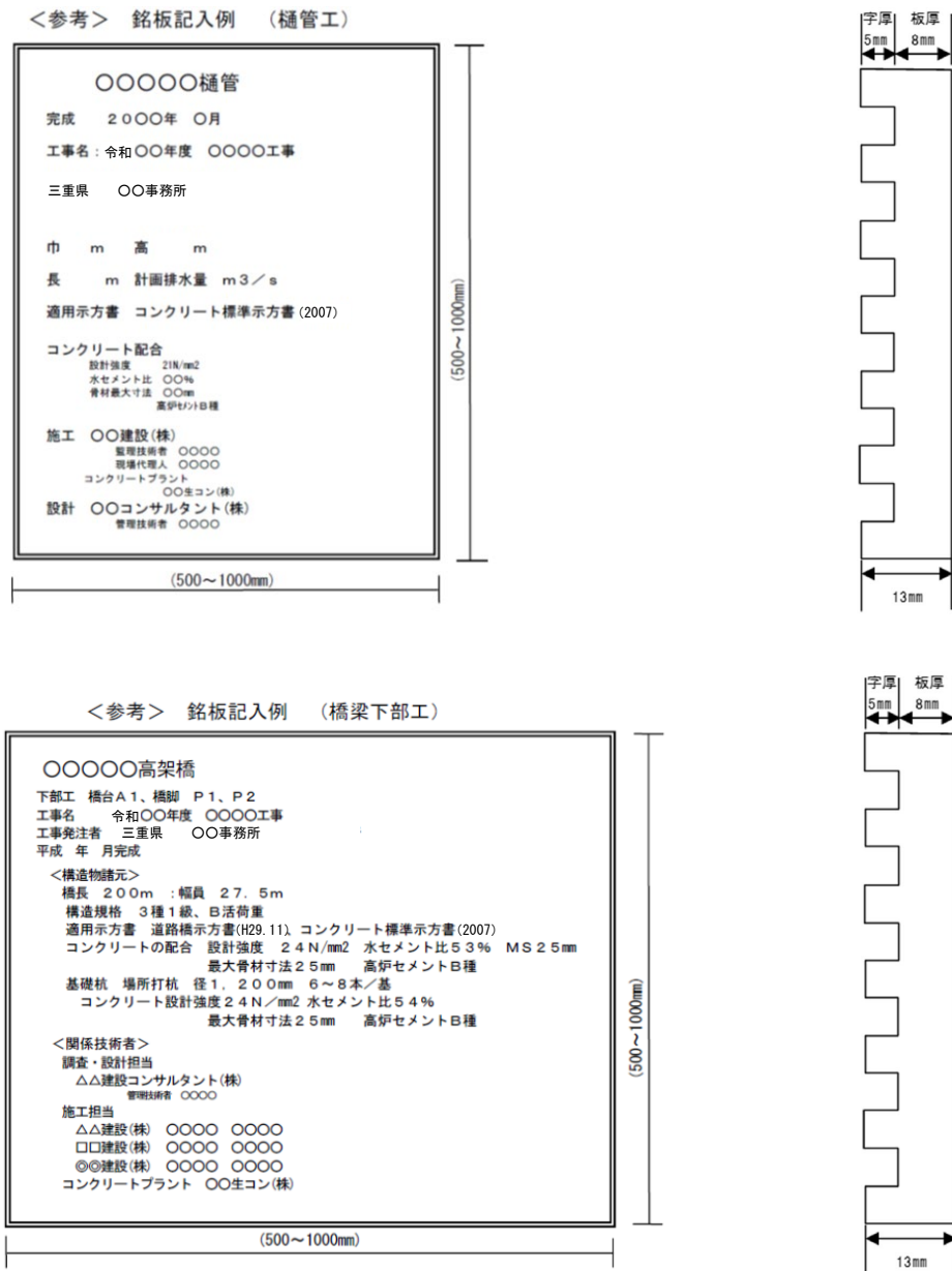
図3-1 銘板記入例
