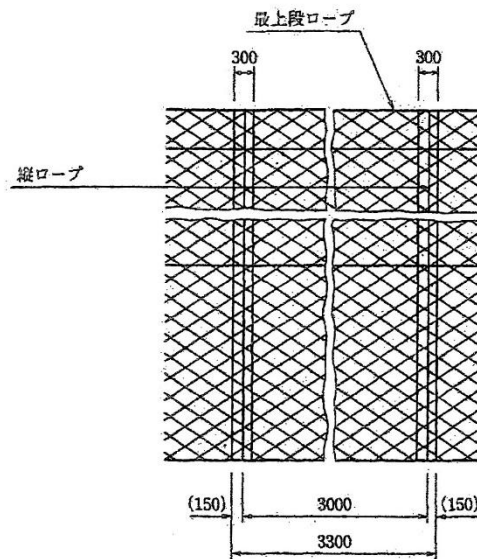
金網重ね詳細図
