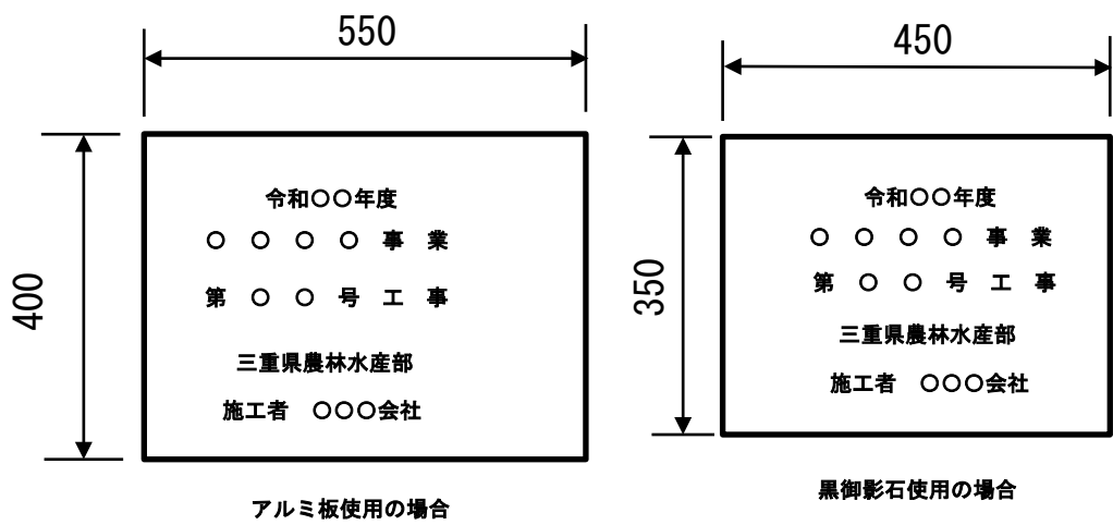
図 4 施工銘板
