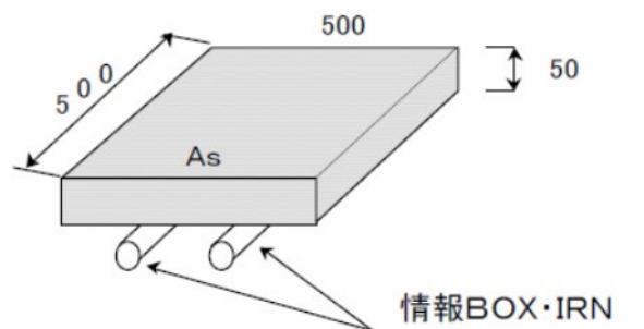
図1-1 試掘標準図
