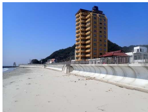
老朽化した堤防の前面に大型波返し護岸（高さを低減）を設置（南知多海岸）
