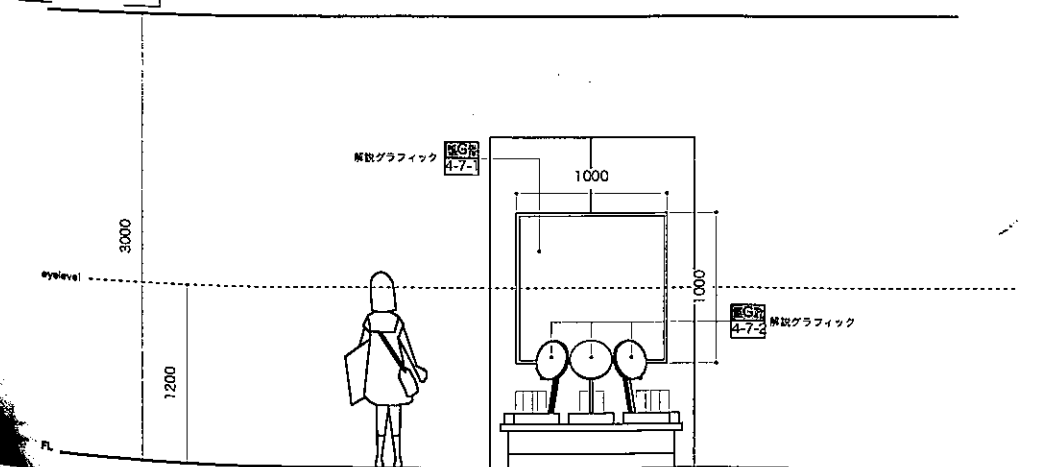
E 立面図
