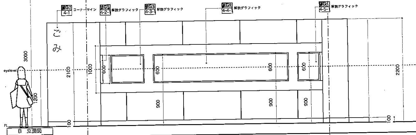
B 立面図
