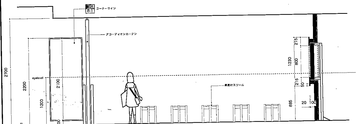
A 立面図
