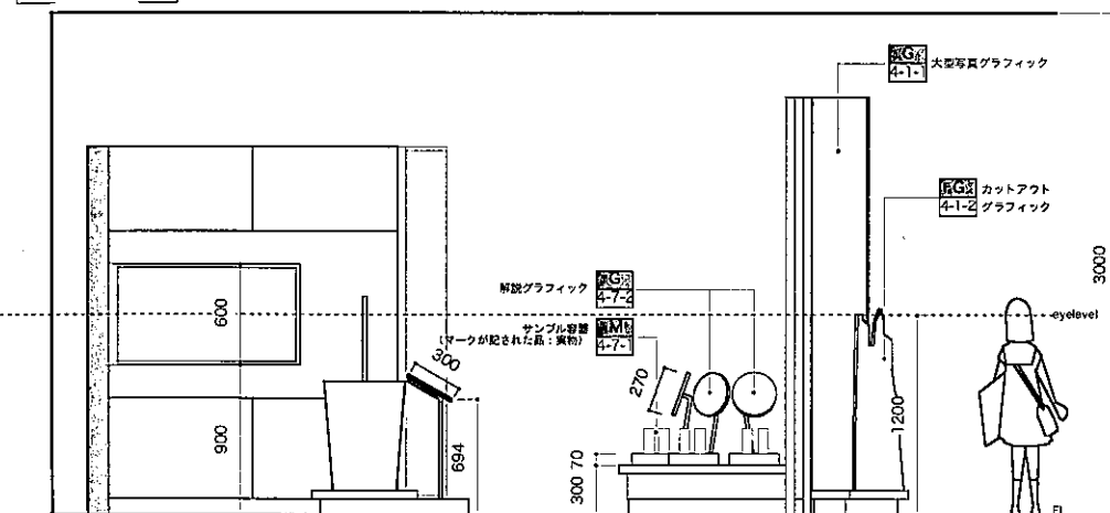
D 立面図
