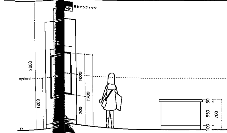
E 立面図
