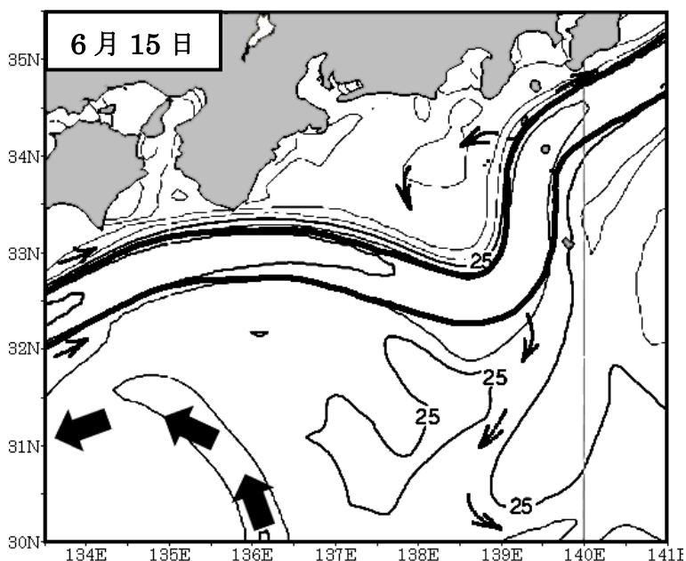
2025/06/15 気象庁 海面水温予想図より [表面水温]
