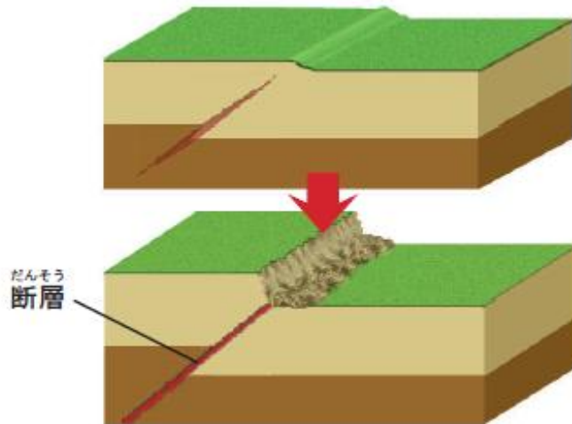
内陸直下型地震の発生メカニズム
