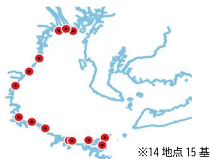
図表 142 伊勢湾において県が設置した ICT ブイ（令和 7 年 3 月時点）
