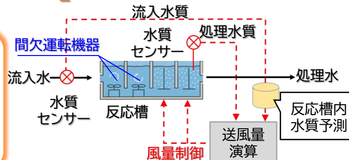
风量制御と間欠運転のイメージ図
