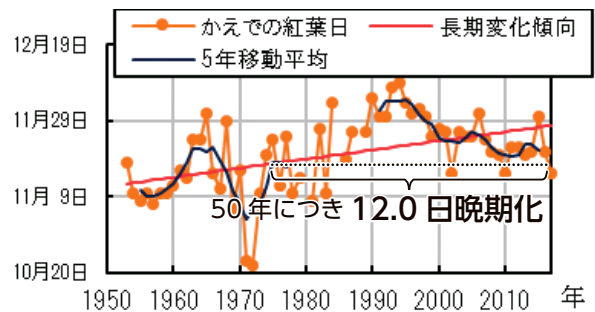
図 3.3-3 津のかえで(イロハカエデ)紅葉日の変化 出典: 津地方気象台からの資料提供
