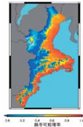
図 3.1-5 ミナミアオカメムシ越冬可能地域予測モデル
