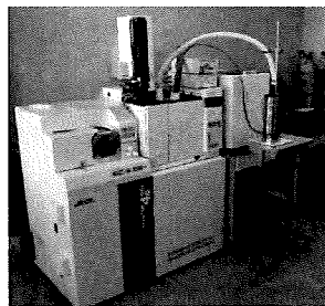
ガスクロマトグラフ質量分析装置 (GC-MS)
