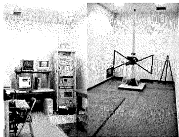
放射ノイズ測定システム
