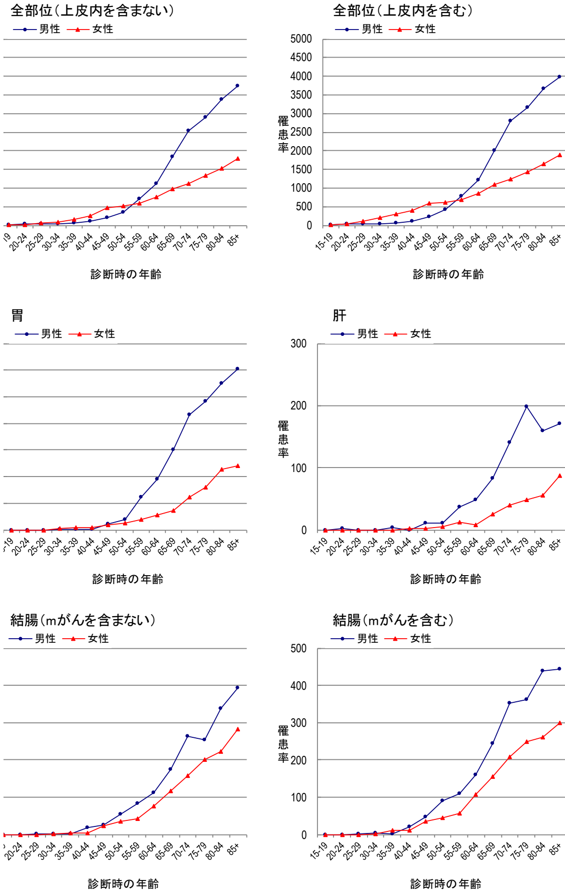
図4 部位別年齢階級別罹患率：人口10万対（表3-A、Bから作成）
