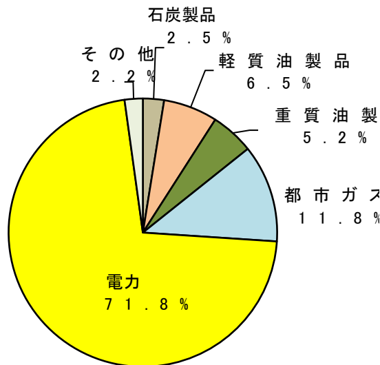
図 13 業務その他部門におけるCO 2 排出量の構成比
