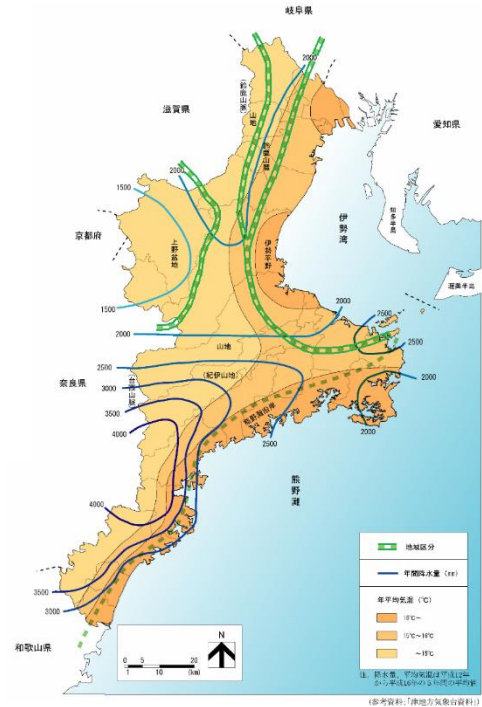
図 28 三重県の気候特性
