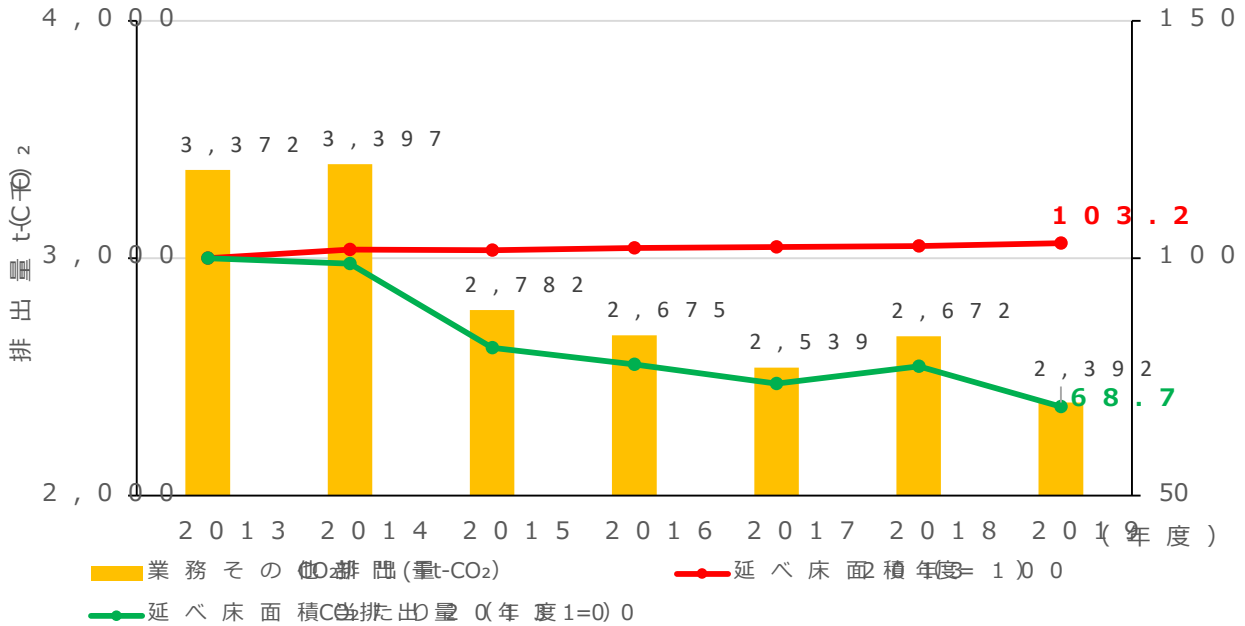
図 12 業務その他部門におけるCO 2 排出量の推移
