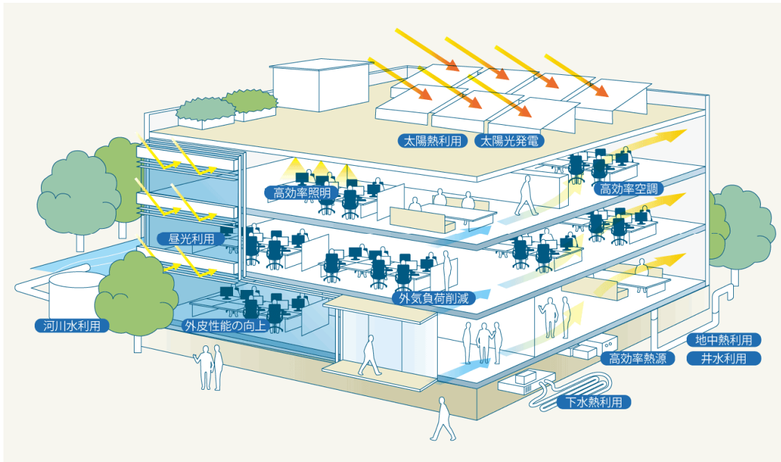
図 23 ZEBの概念図 (イメージ) 出典：資源エネルギー庁ホームページ
