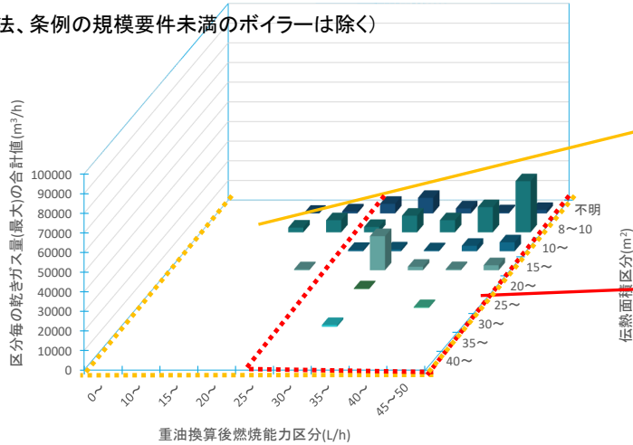
伝熱面積・燃焼能力区分毎の排出ガス量合計 希硫ガス燃料以外
