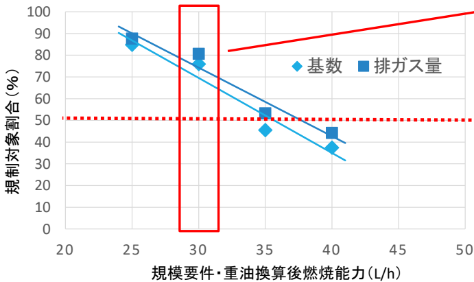
燃焼能力50L/h未満のボイラー中で各規模要件毎の象ボイラーが占める割合(希硫ガス燃料以外)
