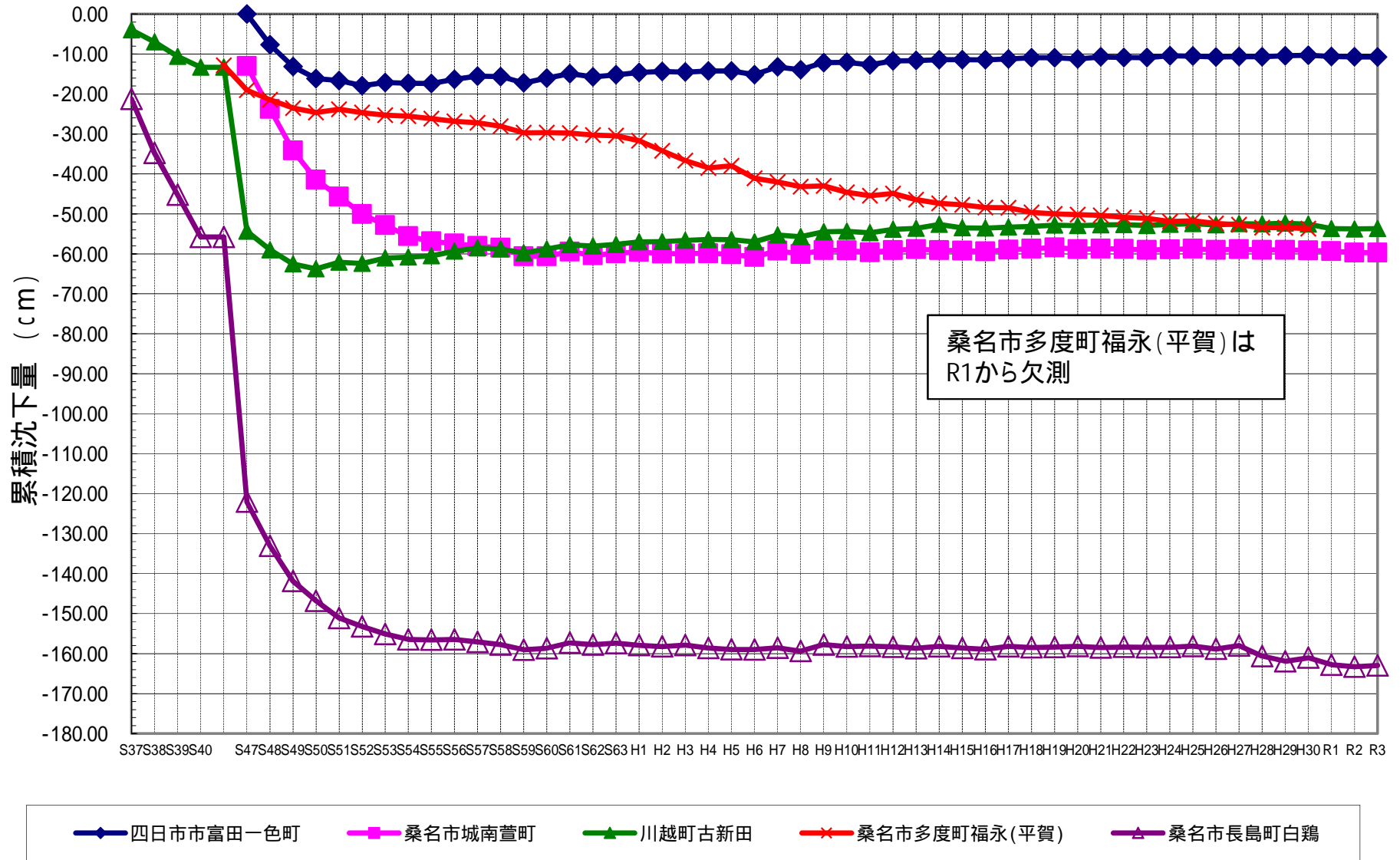
図 - 1 主な水準点の経年変化
