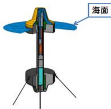
リニア式波力発電（出所：東京大学提供）
