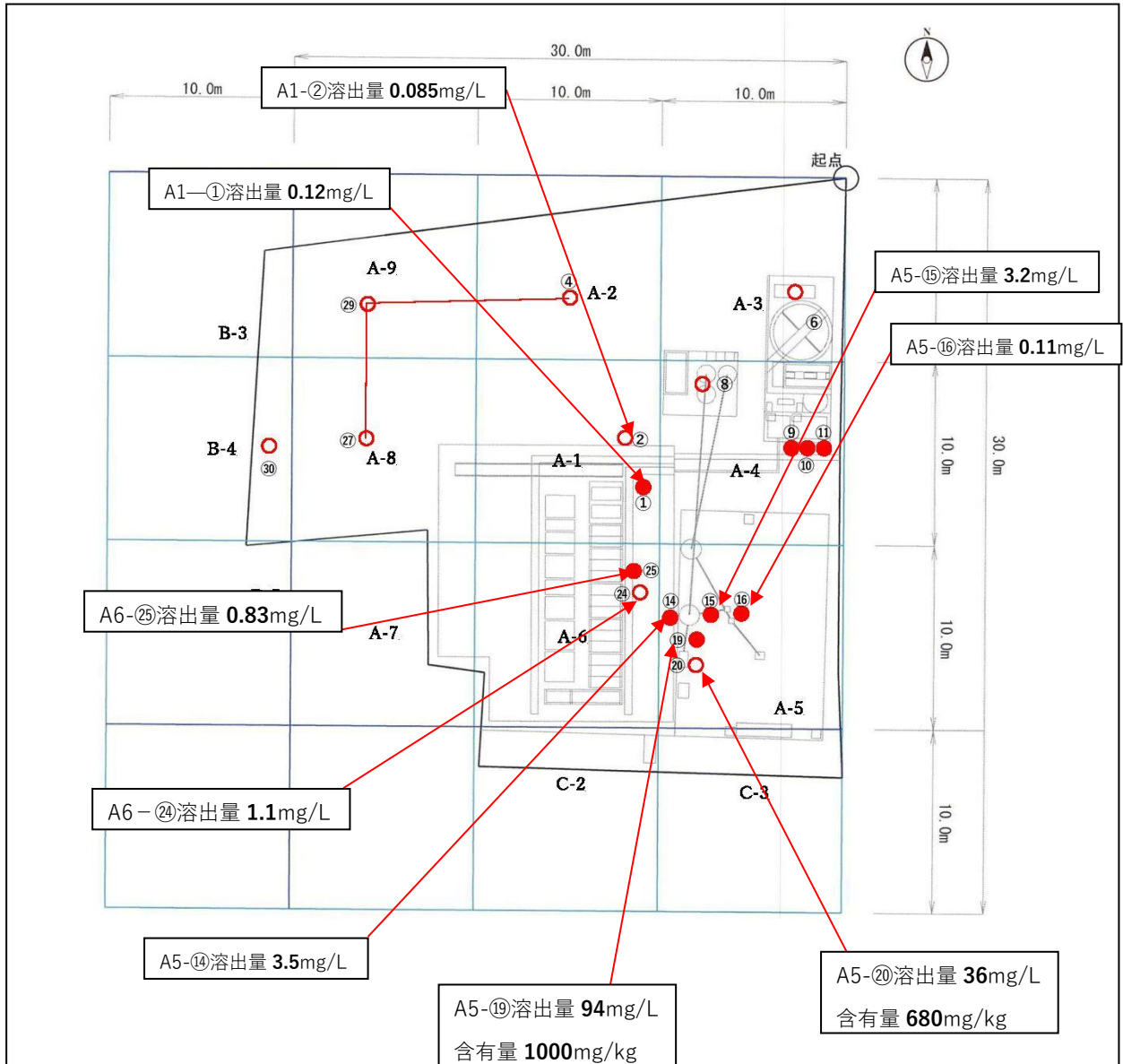
六価クロム分析結果平面図
