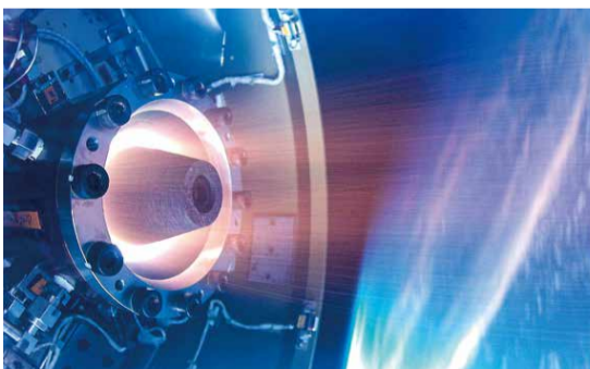
エンジンの気体燃料噴出部分に水谷精機工作所が製作した部品が使用されている。次に打ち上げるロケットにも使用される予定。（写真提供：JAXA、名古屋大学）
