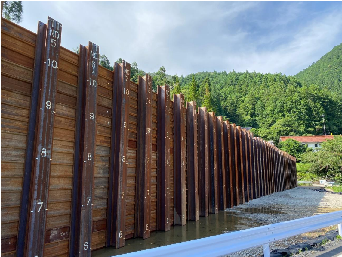
(鋼製山留工)
