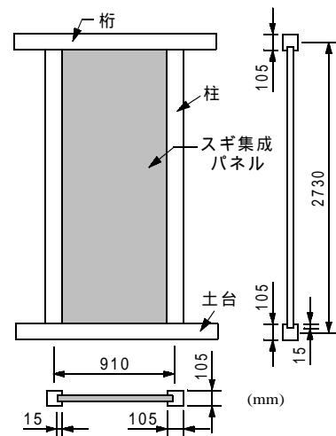
図 - 1 壁試験体図
