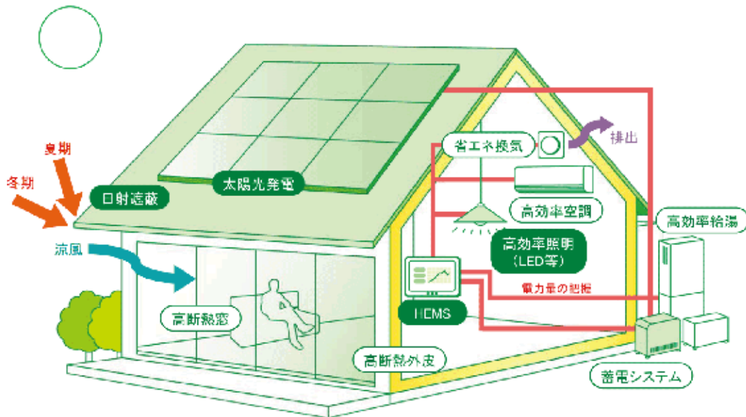
図 18 ZEHの概念図 (イメージ)
