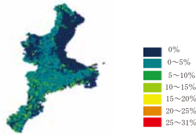
図28 斜面崩壊発生確率の上昇率（2081～2100年と1981～2000年との差）の予測 RCP8.5、MIROC5の例 S-8 温暖化影響・適応研究プロジェクトチームからの提供資料をもとに作成
