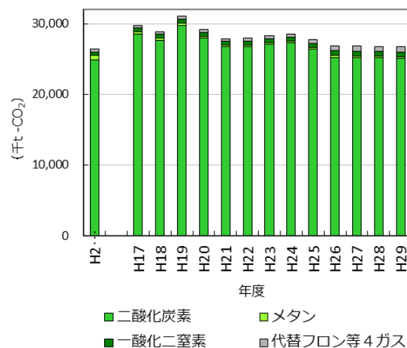
図2-1-1 県域の温室効果ガス排出量の推移
