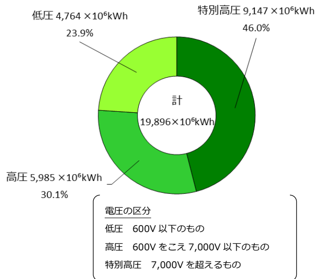
図 2-1-4 三重県の電力需要実績(平成 30(2018)年度)
