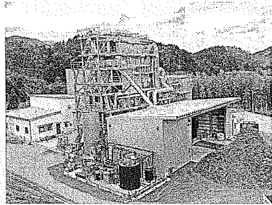
木質バイオマス発電所（松阪市）
