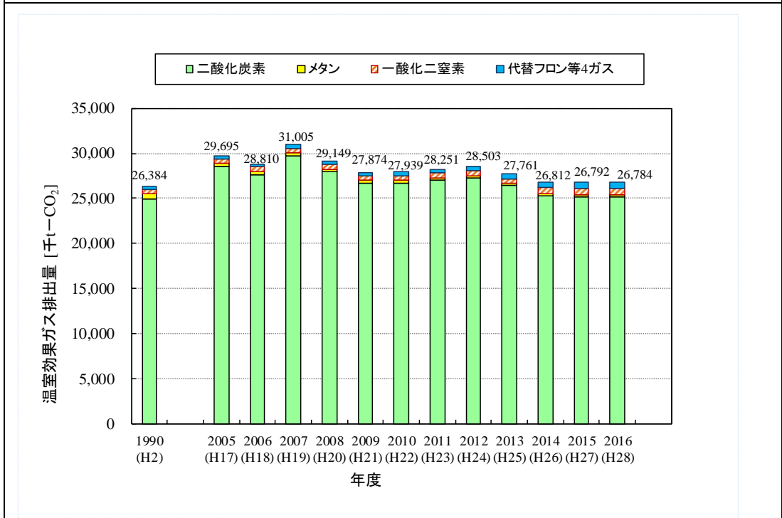
図 1-2 県内の温室効果ガス排出量の推移
