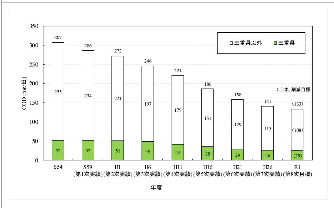
図 4-2 伊勢湾発生汚濁負荷量(COD)の経年変化
