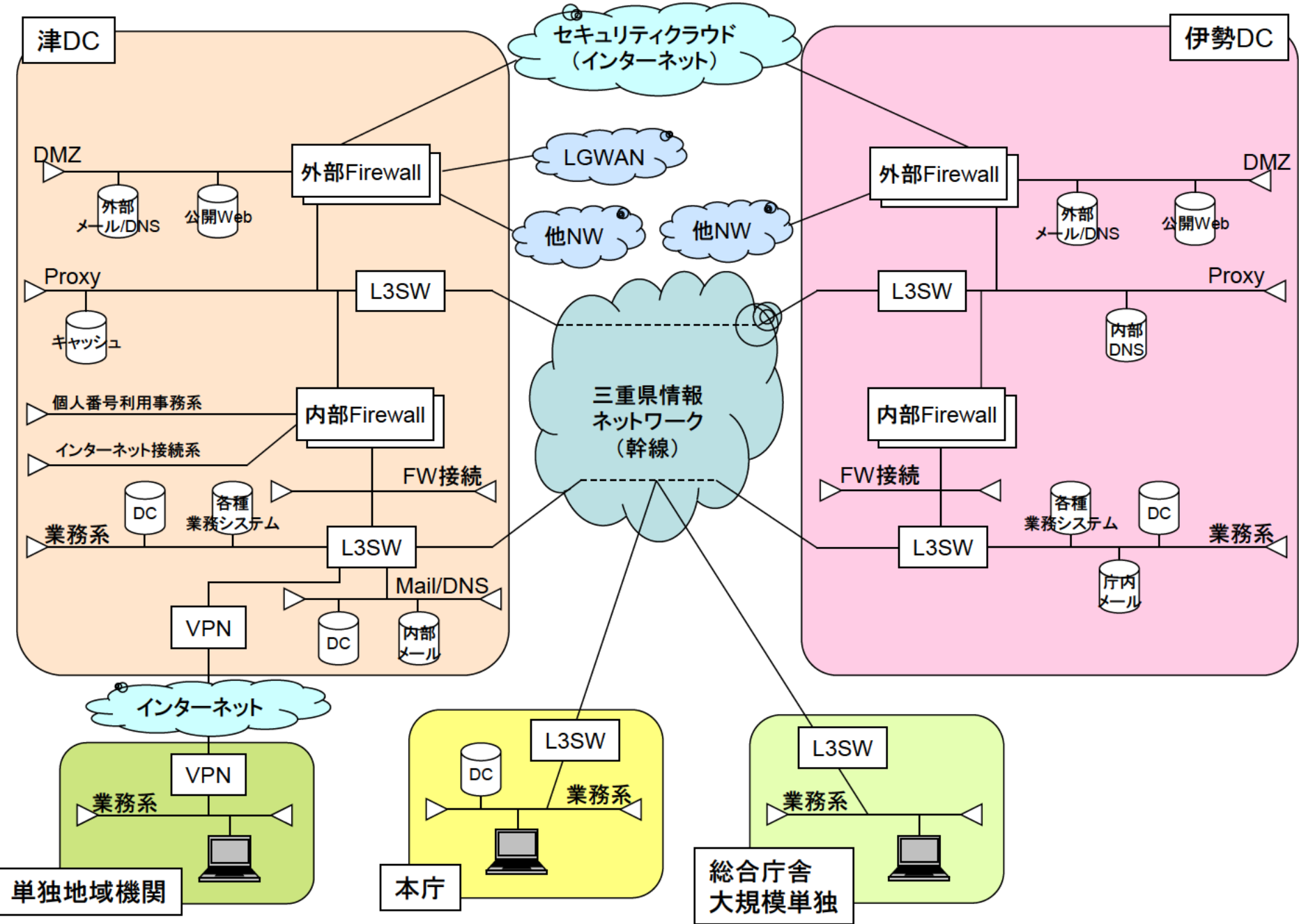
別紙2 三重県行政WAN 論理ネットワーク概要図(現行)
