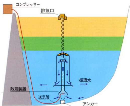
図 3.2-2 比奈知ダムの深層曝気装置 出典:平成 21 年 2 月比奈知ダム定期報告書(案) 概要版(独立行政法人水資源機構)
