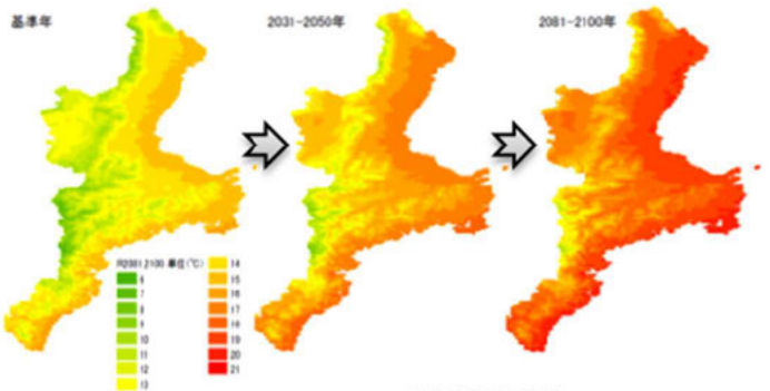
図 4.3-4 三重県の年平均気温の将来予測 (気候予測モデル: MIROC3.2hires, 単位: °C) 出典: 簡易推計ツール(国立環境研究所)に格納されているデータ
