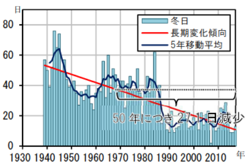
図 2.1-17 尾鷲の冬日の経年変化
