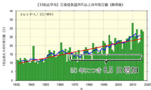
図 2.1-6 日本の熱帯夜の年間日数
