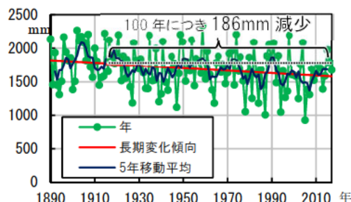
図 2.2-4 津における年降水量の経年変化
