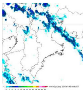
図 2.4-4 レーダーエコー(雨雲レーダー) 出典:2017年1月14日から16日にかけての大雪に関する三重県気象速報(津地方気象台)
