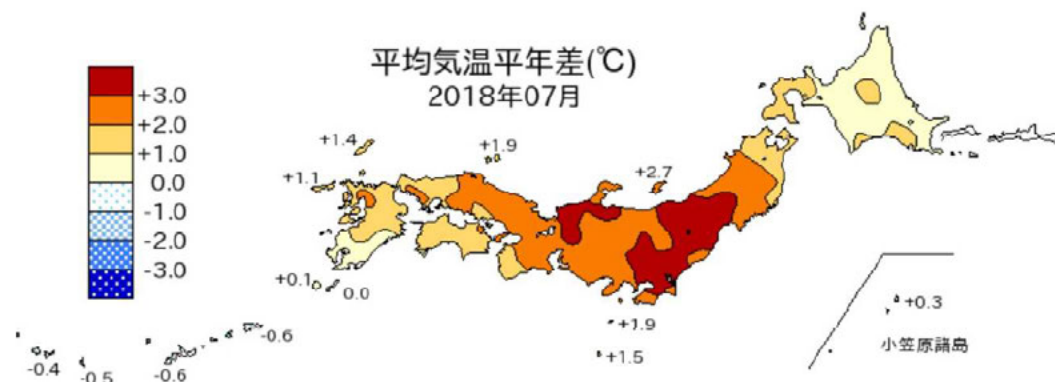
図 2.1-18 2018年7月の平均気温平年差 出典:気象庁Webページ
