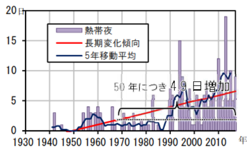
図 2.1-16 尾鷲の熱帯夜の経年変化
