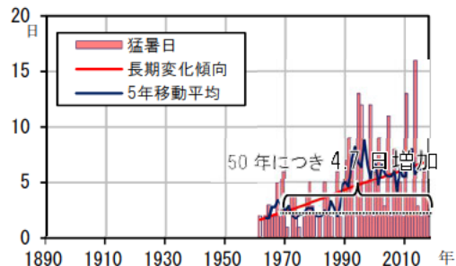
図 2.1-10 津の猛暑日の年間日数
