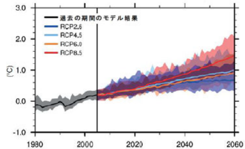
図 4.1-2 世界の海面水温の変化予測 出典:IPCC(2013a) Figure11.19 (気候変動の観測・予測及び影響評価統合レポート2018(環境省)) 1986年から2005年の平均値に対する海面水温の変化
