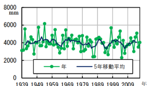
図 2.2-6 尾鷲における年降水量の経年変化
