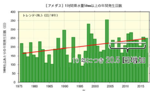
図 2.2-3 1 時間降水量 50 mm 以上の年間発生回数の経年変化 出典:気候変動監視レポート 2017 (気象庁)より作成 棒グラフ(緑):国内のアメダスによる観測を 1000 地点あたりに換算した各年間発生回数の平均値 直線(赤):長期変化傾向
