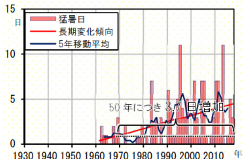
図 2.1-15 尾鷲の猛暑日の経年変化
