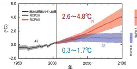
図 4.1-1 2081~2100年における年平均地上気温の変化予測 出典:IPCC AR5 WG1 SPM.7(a) (気象庁 Web ページより作成) 1986年から2005年の平均値に対する平均気温の変化
