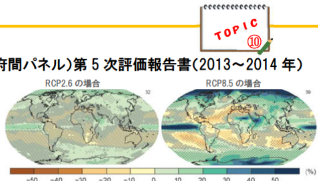
図 4.3-8 年平均降水量変化(1986~2005年平均と2081~2100年平均の差) 出典:IPCC AR5 WG1 SPM 図 SPM.8(b) (気象庁 Web ページ)
