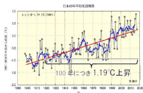
図 2.1-3 日本の年平均気温偏差の経年変化 出典: 気候変動監視レポート 2017(気象庁)より作成
