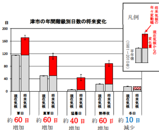
図 4.3-2 夏日、真夏日、猛暑日、熱帯夜、冬日の日数の変化予測(RCP8.5)
