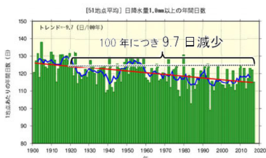
図 2.2-2 日降水量 1.0mm 以上の年間日数の経年変化 出典:気候変動監視レポート 2017 (気象庁)より作成 棒グラフ(緑):国内 51 地点での日降水量 1.0mm 以上の年間日数の平均値 折れ線(青):5 年移動平均 直線(赤):長期変化傾向
