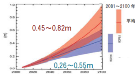
図 2.4-2 21 世紀にわたる世界平均海面水位の上昇予測 (1986~2005 年平均との比較) 出典：IPCC AR5 WG1 SPM.9(気象庁 Web ページより作成)
