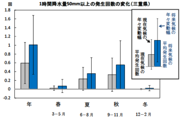
図 4.3-6 県内の短時間強雨(1時間降水量50mm以上)の変化予測(RCP8.5) 出典:津地方気象台からの提供資料
