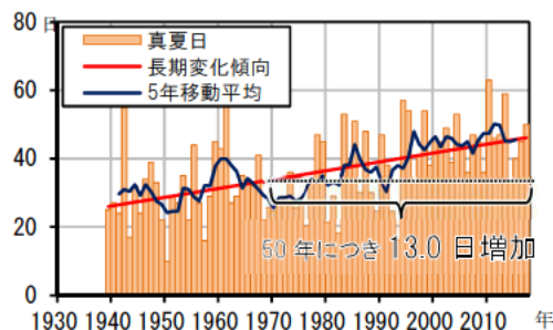
図 2.1-14 尾鷲の真夏日の経年変化
