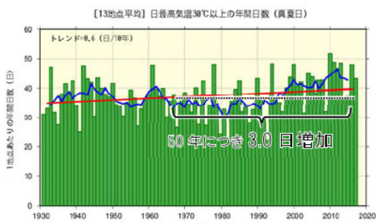
図 2.1-4 日本の真夏日の年間日数
