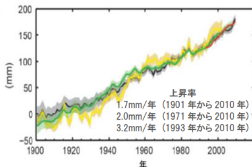
図 2.4-1 世界海面水位の経年変化 出典：気候変動の観測・予測及び影響評価統合レポート 2018(環境省)より作成 1900年から1905年の平均値を基準とした世界平均海面水位
