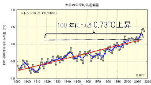
図 2.1-1 世界の年平均気温偏差の経年変化 出典: 気候変動監視レポート 2017(気象庁)より作成
