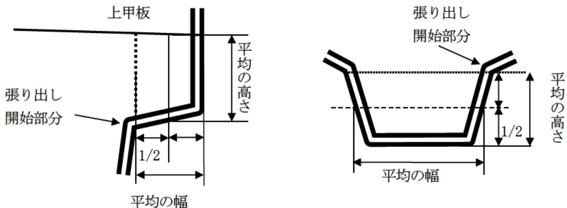
張り出し部の平均の幅、平均の高さ
