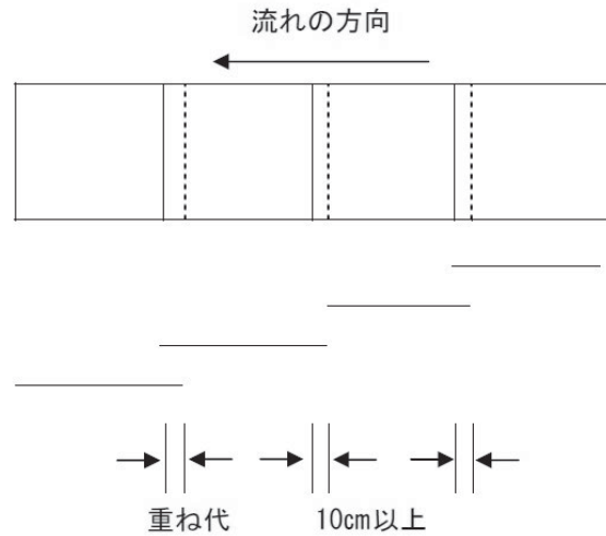
図1-1 吸出し防止シートの重ね代
