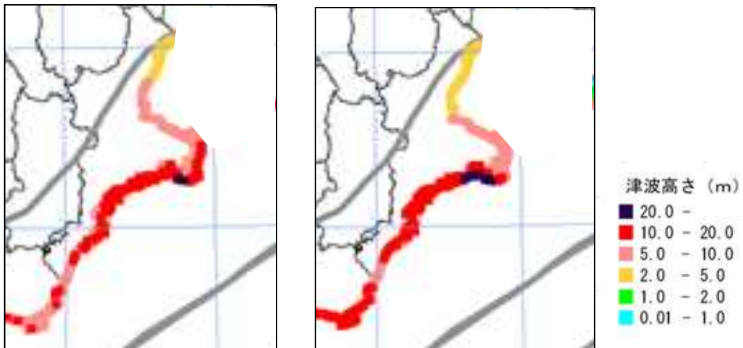
理論上最大モデルの津波（ケース①：左図、ケース⑦：右図）の津波高（満潮水位 地盤変動量考慮）
