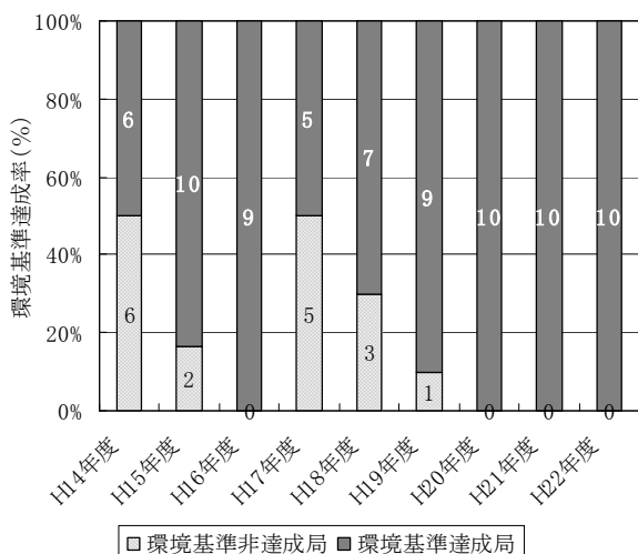
図(2) ① SPM 環境基準達成状況の推移 (対策地域内 一般局)
