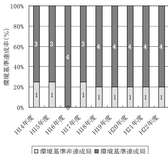
参照図(1) 対策地域内測定局の二酸化窒素環境基準達成状況の推移 (グラフ内の数字は測定局数を示す。)
