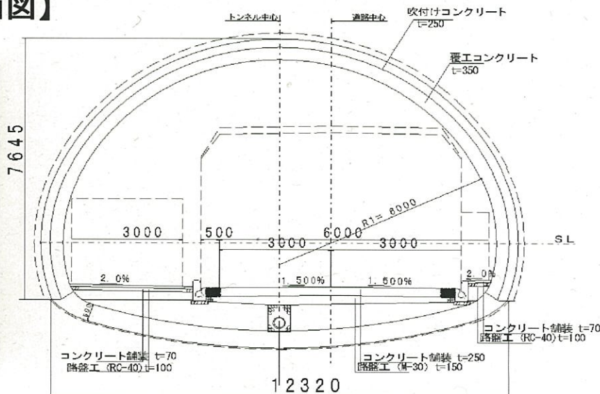
標準断面図 (DⅢa-1)
