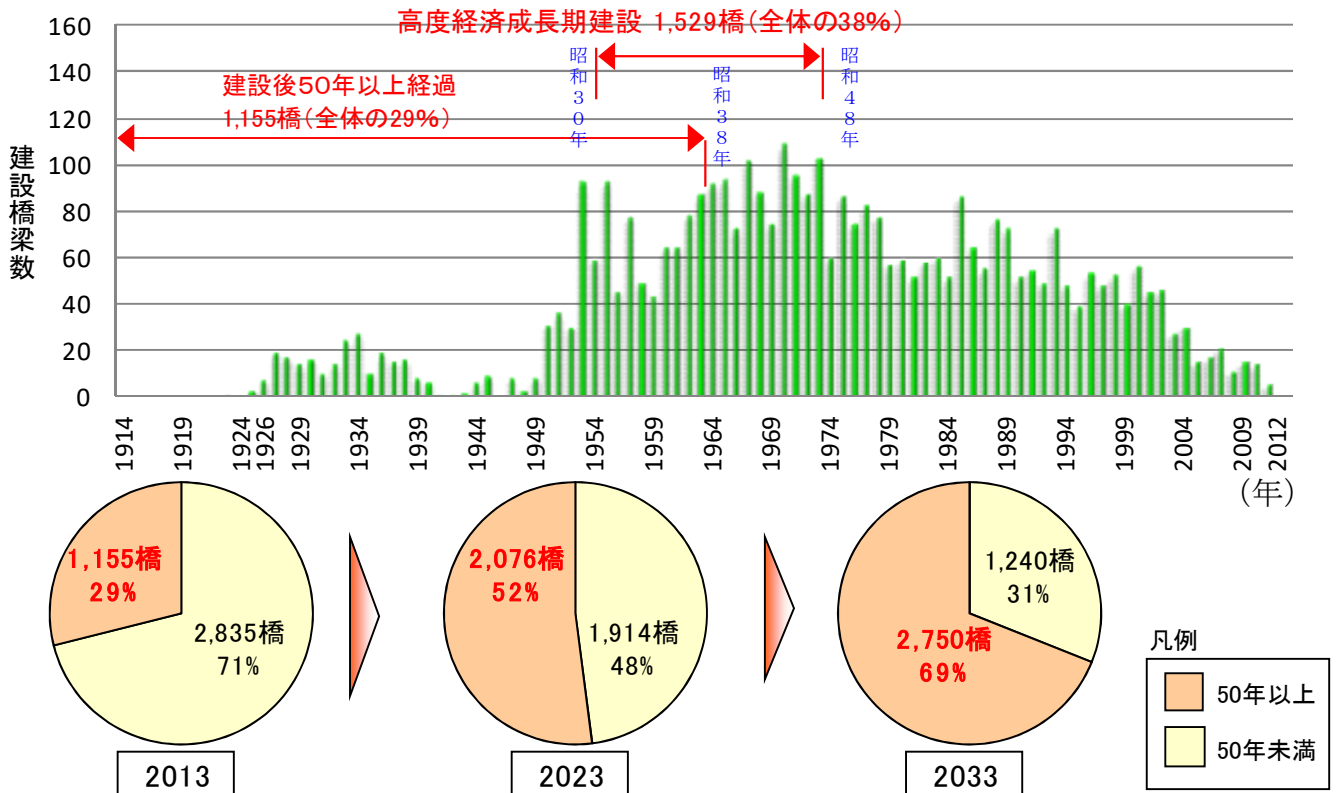
第14図 橋梁の老朽化状況 ..... 本冊 6 ページ
