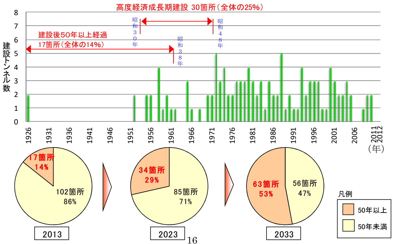
第15図 トンネルの老朽化状況 ..... 本冊 6 ページ
