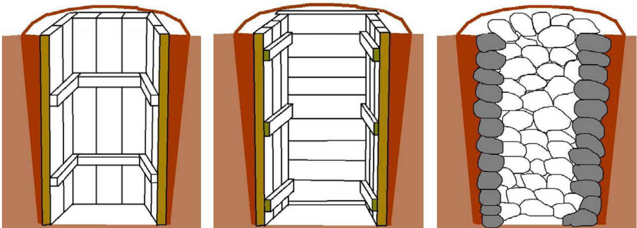
縦・横板組横棧どめ
