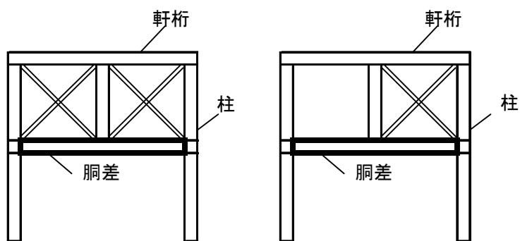
片筋交いの場合も同様
