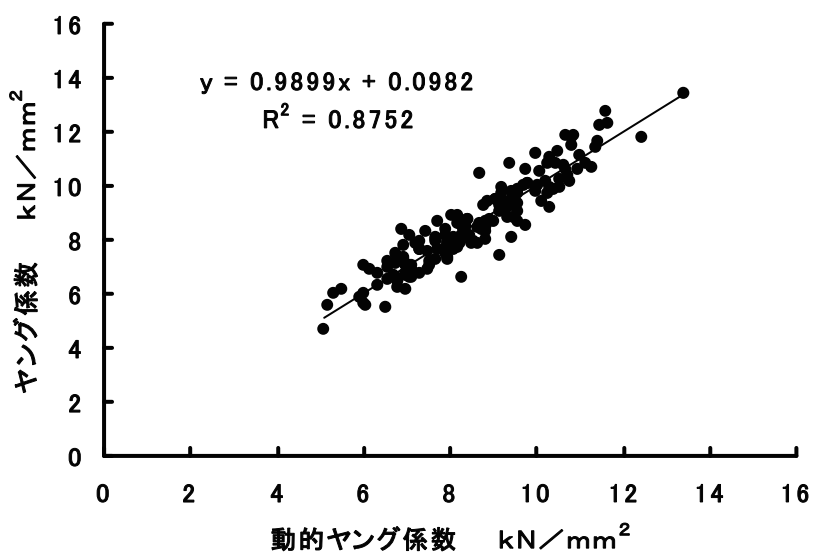
図 5 ヤング係数の相関(スギ)
