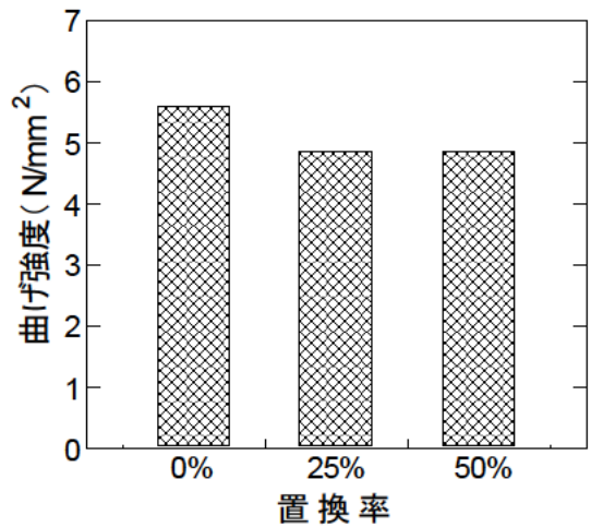
図4 曲げ強度
