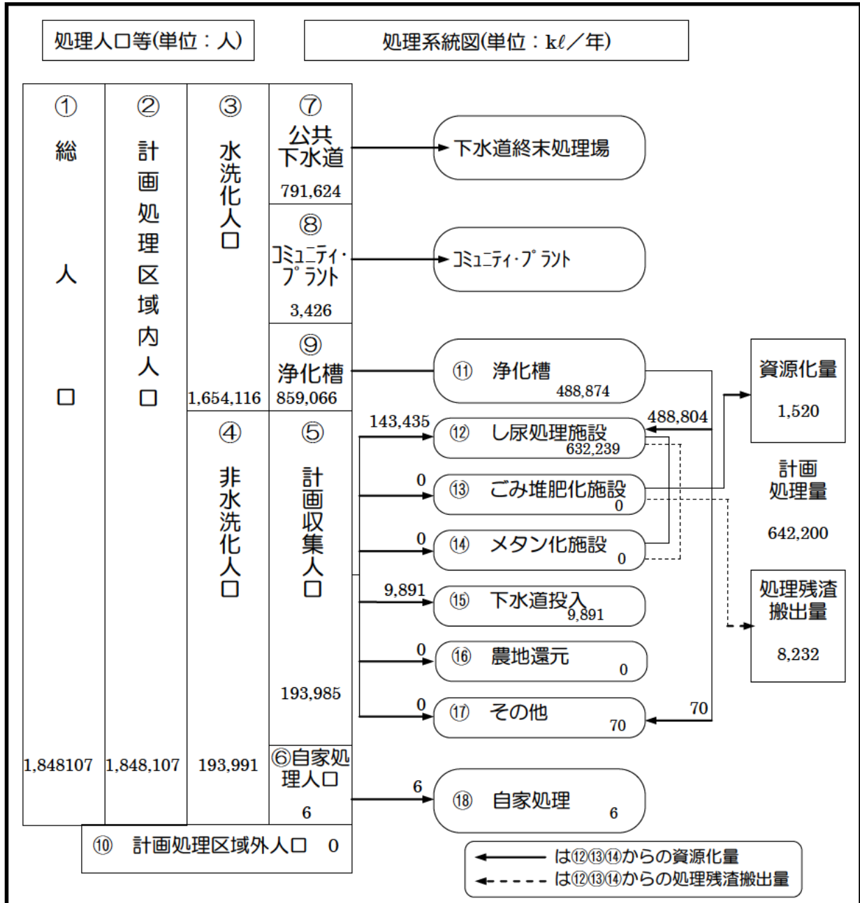
資料7-11 し尿処理のフロー図（平成23年度）
