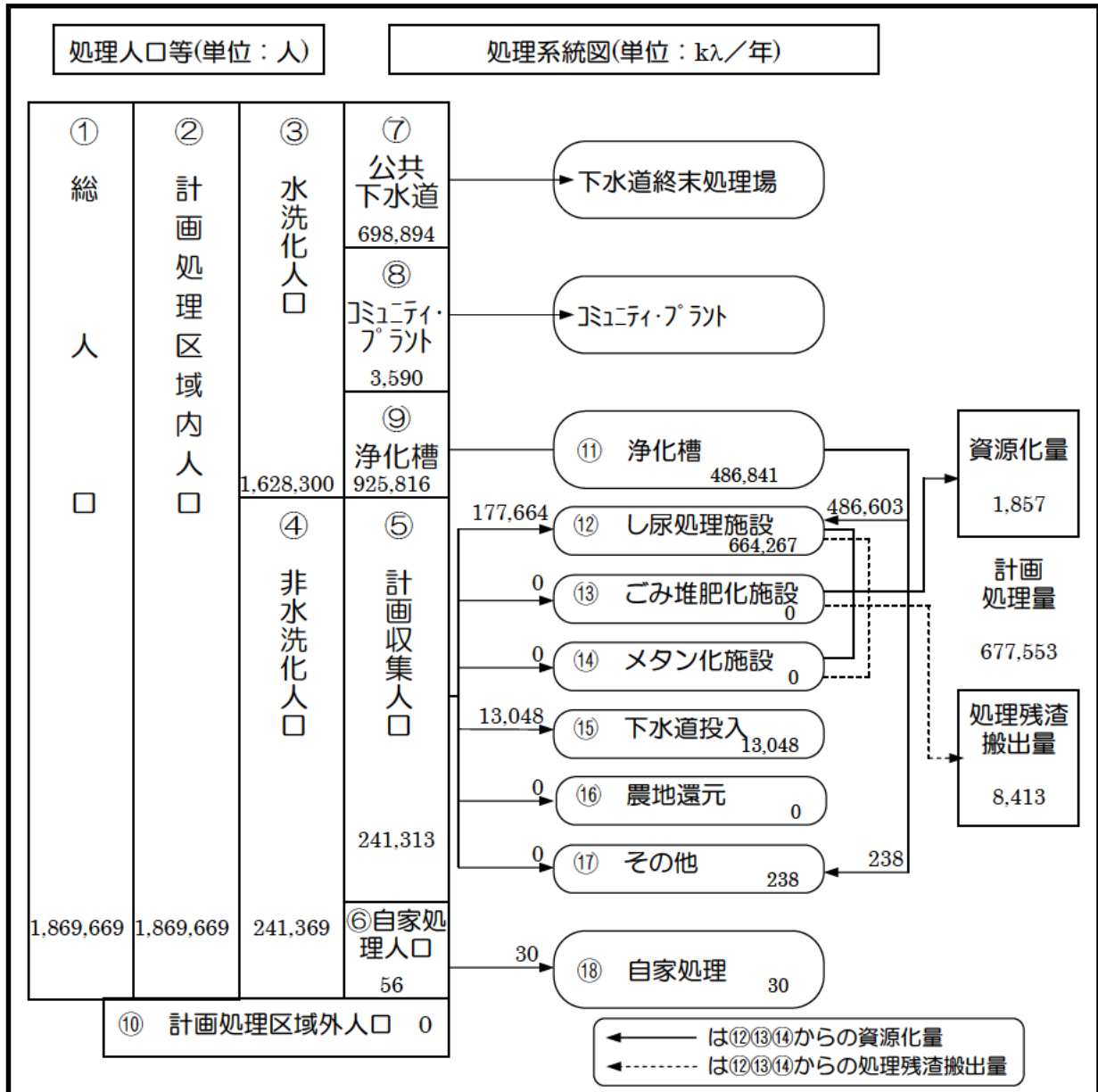
資料7-11 し尿処理のフロー図（平成20年度）
