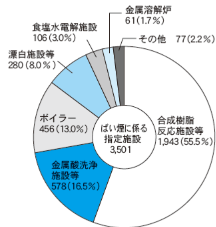
図 1-3-10 ばい煙に係る指定施設の種別内訳 (平成14年3月31日現在)
