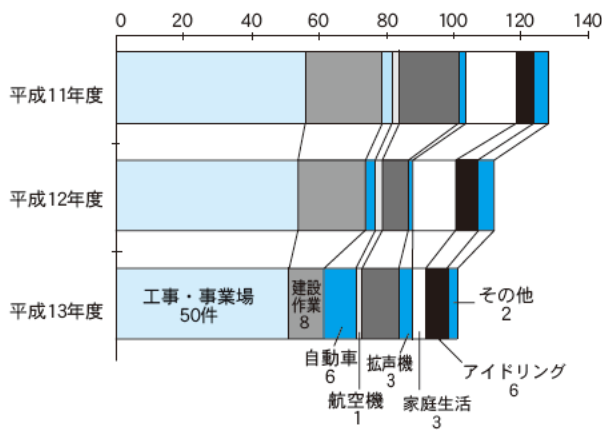
図 1-3-13 騒音苦情の発生源別の申立状況
