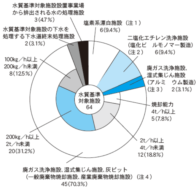
図 1-3-9 水質基準対象施設の種別内訳 (平成14年3月31日現在)
