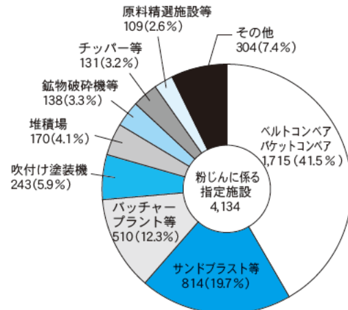
図 1-3-11 粉じんに係る指定施設の種別内訳 (平成14年3月31日現在)
