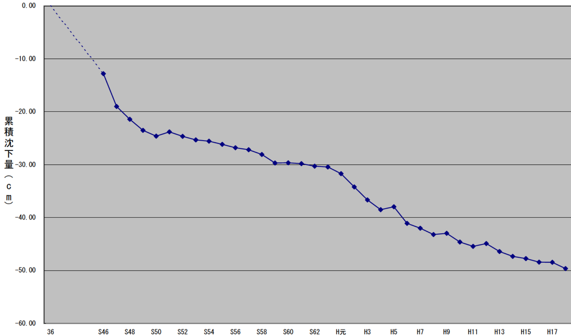
図一3 年間1cm以上の沈下を示した点の経年変化 桑名市多度町福永(平賀)
