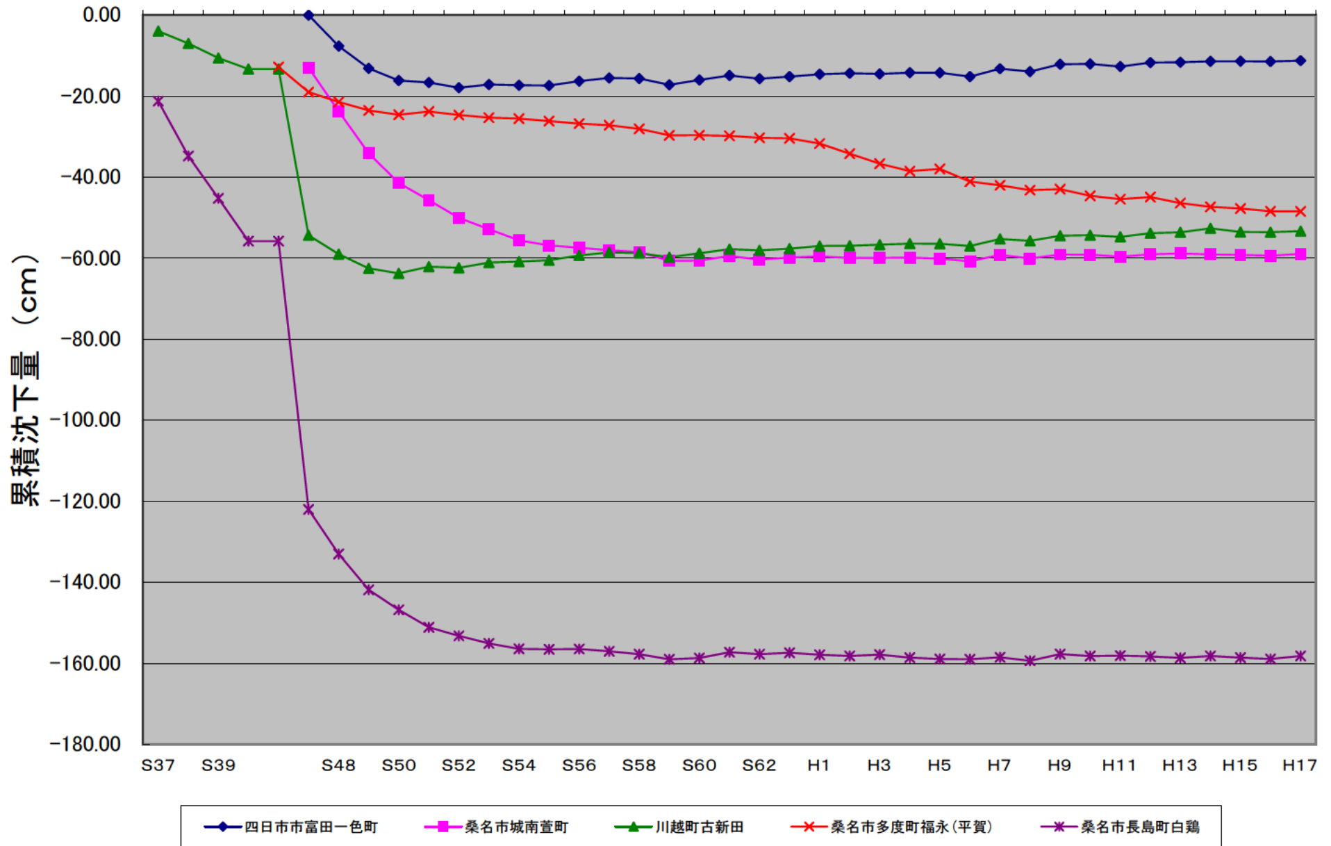
図-1 主な水準点の経年変化
