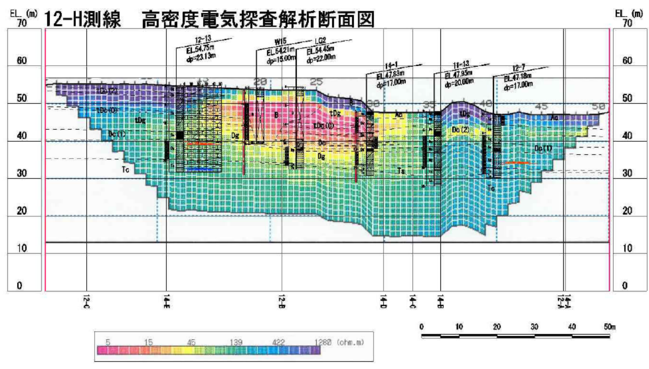
図一 電気探査 12-H 測線沿い地質および帯水層区分断面図
