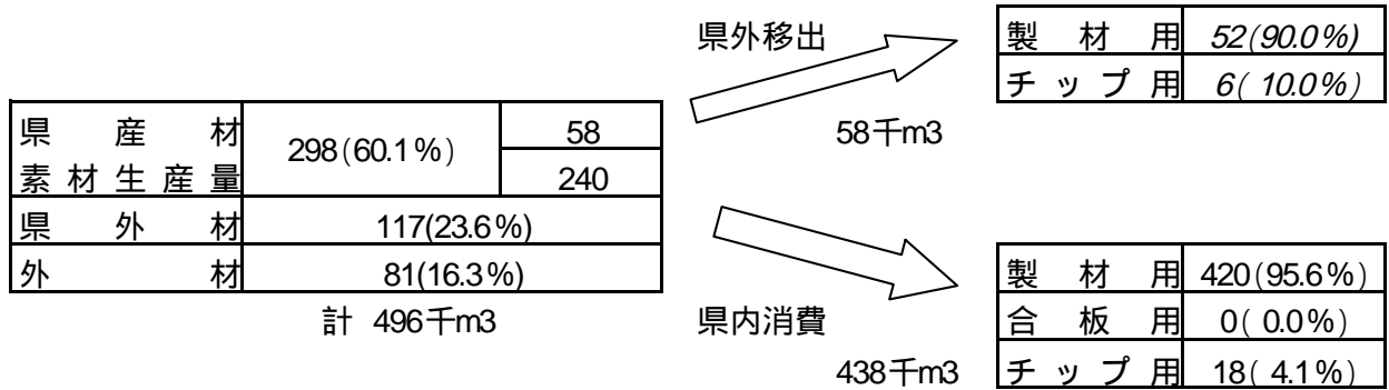
素材の流れ
