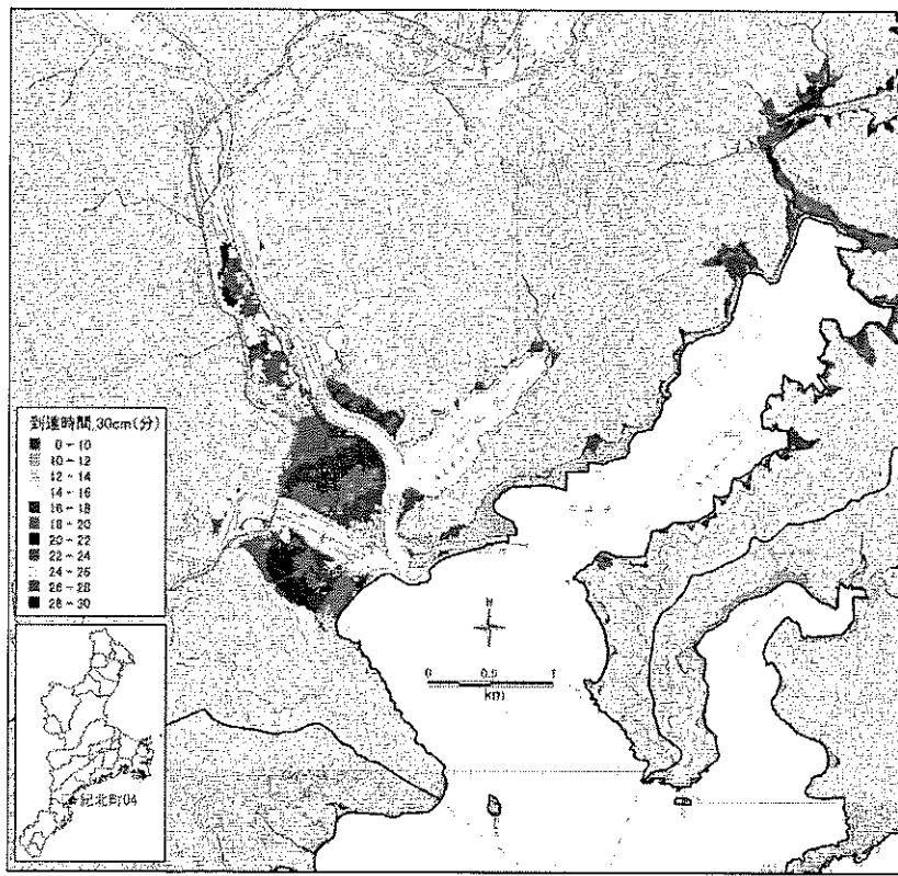
津波浸水深 30cm 到達予測時間分布図 (紀北町 04)
