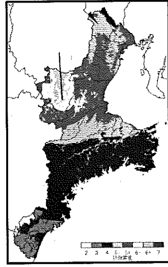
頓宮断層
