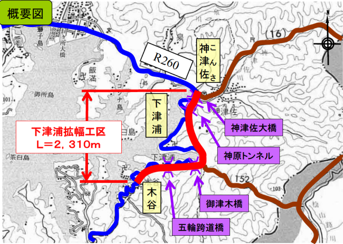
①現道(事業着手当時)
