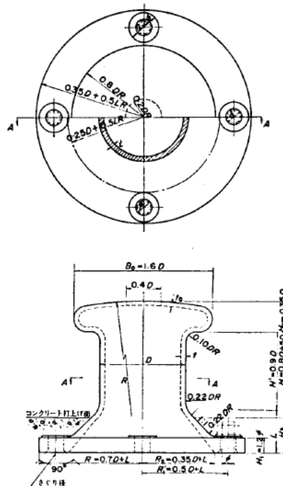
図2-1 直柱の標準寸法と設計けん引力
