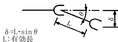
許容曲げ角度と偏位 (S II形)
