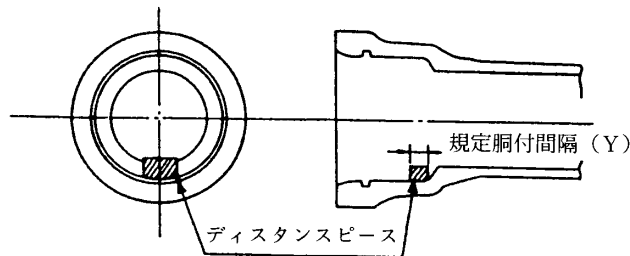
胴付間隔
