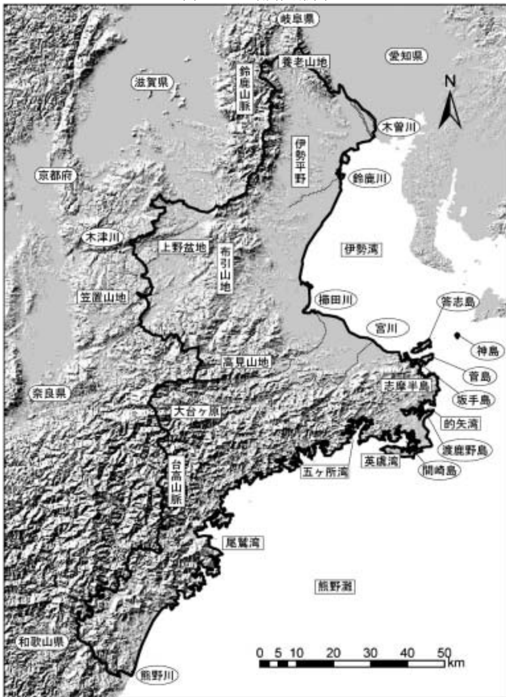
図1-2 概略地形図
